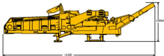
HG6000E II 標準仕様(単位mm)
