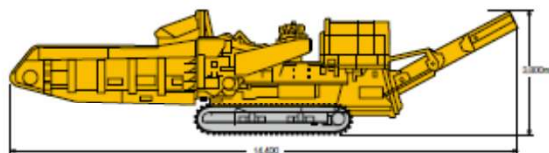
HG6000TX II 標準仕様(単位mm)
