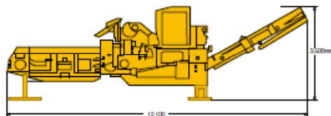
HG4000E II 標準仕様(単位mm)
