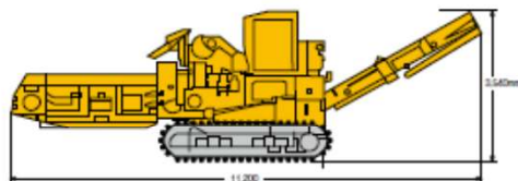
HG4000TX II 標準仕様(単位mm)
